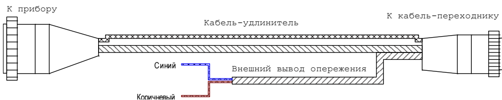
Рисунок 18. Кабель-удлинитель
